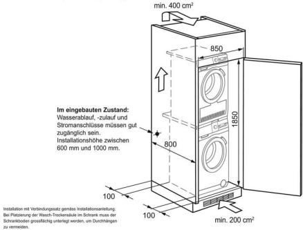
Belüftungsbeispiel für Wasch-Trockensäule, Schrankinbau, Tür muss bei Betrieb geöffnet sein (Belüftung in Möbel integriert)
